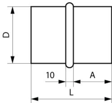
Ниппель внутренний
